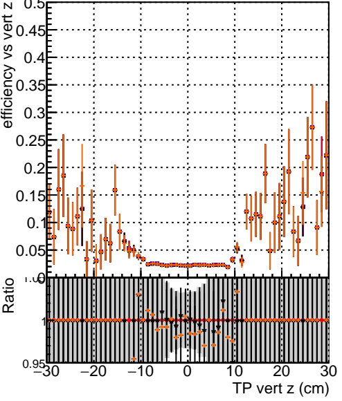
Efficiency vs vert r Legend: - Blue square: DQM_original_originalvector_1000evt - Red circle: DQM_original_1000evt - Black star: DQM_fitted4_1000evt - Orange triangle: DQM_fit_nocpe_1000evt
