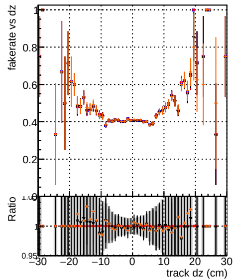
Fake rate vs d Legend: DGM original DGM original+vector_1000evt DGM fit 1000evt DGM fit nocpe_1000evt
