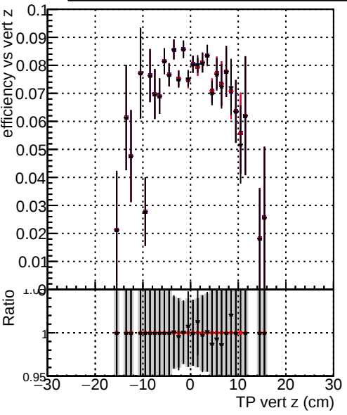
Efficiency vs vert z Legend: DQM_original_originalvector_1000evt DQM_original_1000evt DQM_fitted4_1000evt
