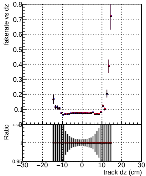
Fake rate vs dz — DOM original 1000evt — DOM original 1000evt — DOM fitted 1000evt
