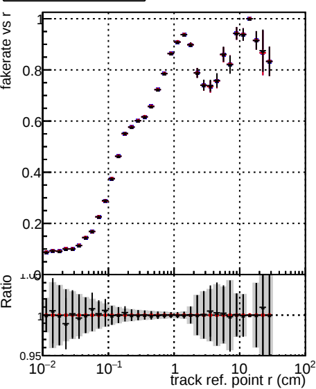
Fake rate vs verpos Legend: —•— DQM_original_originalvector_1000evt —•— DQM_original_1000evt —•— DQM_fitted4_1000evt
