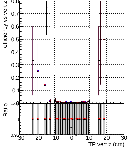
Efficiency vs vert z —●— DQM_original_originalvector_1000evt —●— DQM_original_1000evt —●— DQM_fitted4_1000evt
