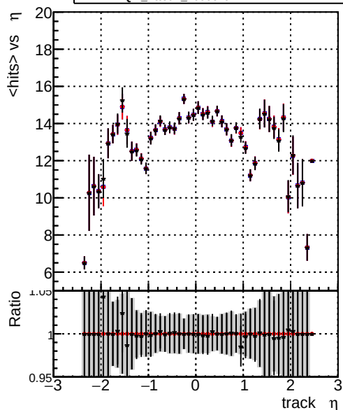
mean hits vs \eta — DQM_original_originalvector_1000evt — DQM_original_1000evt — DQM_fitted4_1000evt
