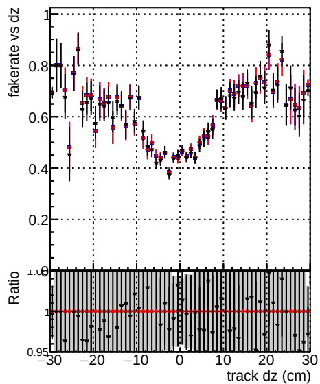
Fake rate vs dz — DOM original 1000evt — DOM original 100evt — DOM fitted 1000evt
