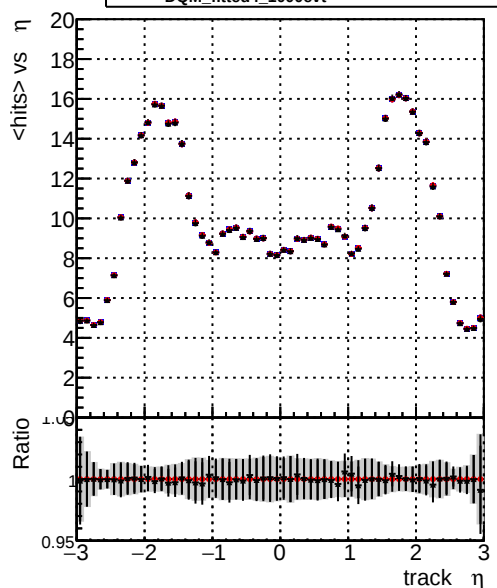
mean hits vs \eta — DQM_original_originalvector_1000evt — DQM_original_1000evt — DQM_fitted4_1000evt
