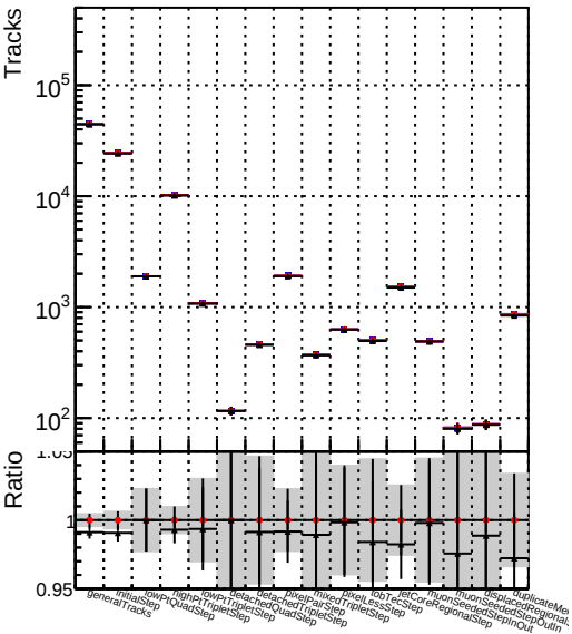
DQM_original_originalvector_1000evt
