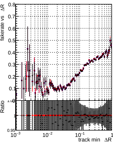
Fake rate vs \Delta R(\text{track, jet}) Legend: DQM original originalvector_1000evt DQM original 1000evt DQM fitted4 1000evt
