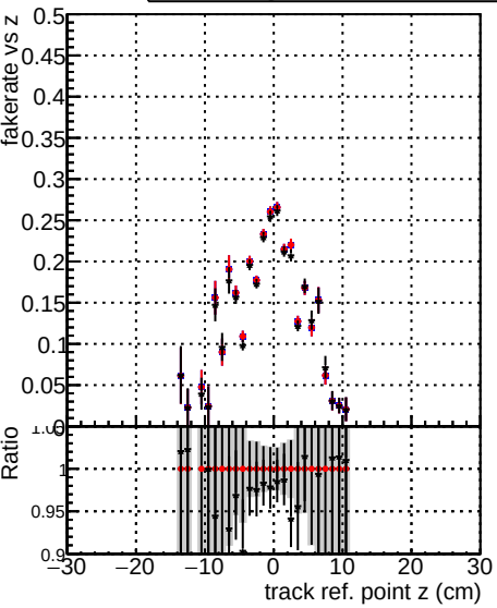
Fake rate vs v DOM original originalvector_1000evt DOM original 1000evt DOM fitted4 1000evt
