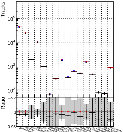
DQM_original_originalvector_1000ev
