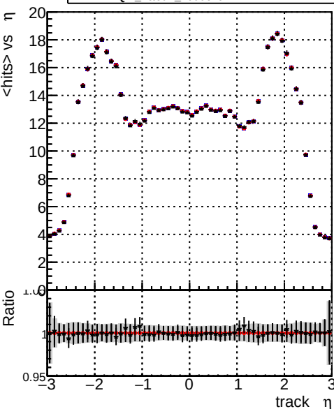
mean hits vs \eta — DQM_original_originalvector_1000evt — DQM_original_1000evt — DQM_fitted4_1000evt
