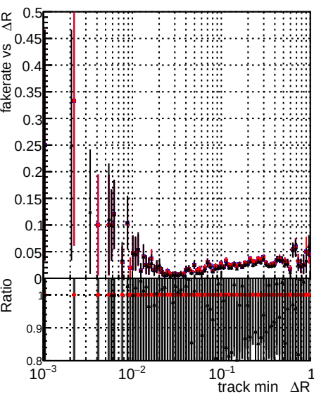
Legend: DQM original originalvector_1000evt, DQM original 1000evt, DQM fitted4 1000evt
