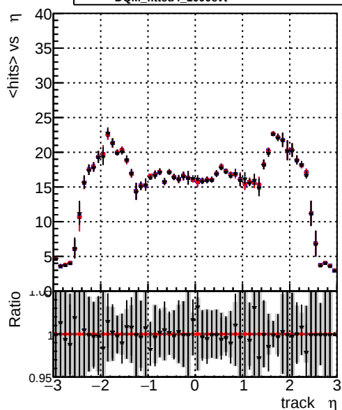
mean hits — DQM_original_originalvector_1000evt — DQM_original_1000evt — DQM_fitted4_1000evt
