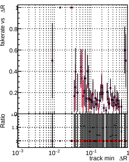
Legend: - \Delta R original originalvector_1000evt - \Delta R original_1000evt - \Delta R fitted4_1000evt
