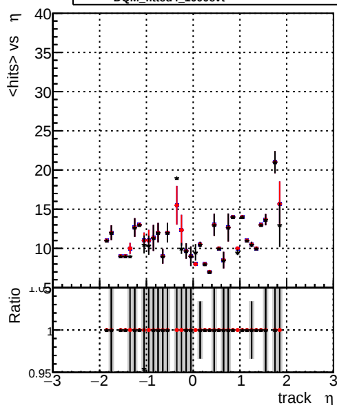
mean hits — DQM_original_1000evt — DQM_fitted4_1000evt
