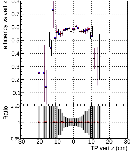
Efficiency vs. TP vert z (cm) Legend: - —•— DQM_original_originalvector_1000evt - —•— DQM_original_1000evt - —•— DQM_fitted4_1000evt
