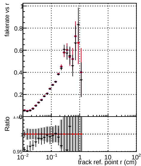
—•— DQM original originalvector_1000evt —•— DQM original 1000evt —•— DQM fitted4 1000evt
