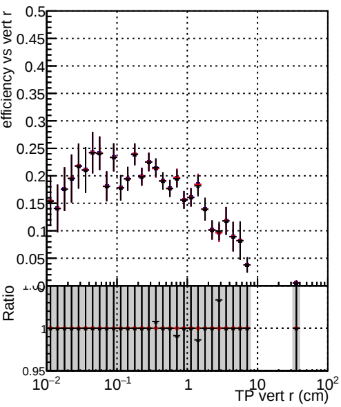
Efficiency vs TP vert r (cm) Legend: DQM_original_originalvector_1000evt DQM_original_1000evt DQM_fitted4_1000evt
