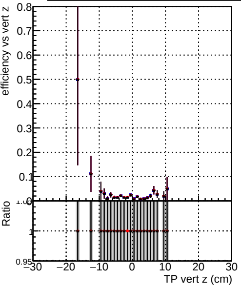
Efficiency vs TP vert z (cm) Legend: DQM_original_originalvector_1000evt DQM_original_1000evt DQM_fitted4_1000evt
