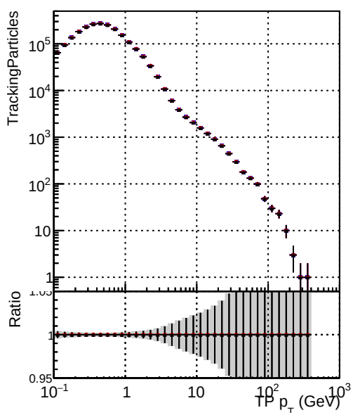
—•— DQM_original_originalvector_1000evt —•— DQM_original_1000evt —•— DQM_fitted4_1000evt
