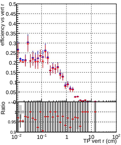
Efficiency vs TP vert r (cm) Legend: DQM_original_1000evt DQM_fitted4_1000evt
