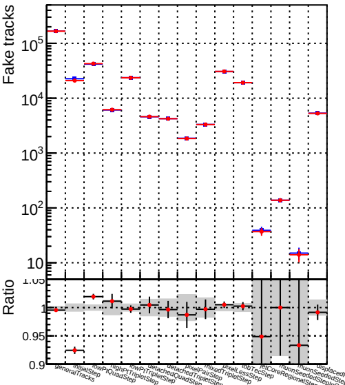
Number —●— DQM_fitted4_1000evt
