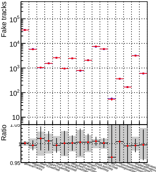
Number —●— DQM_fitted4_1000evt
