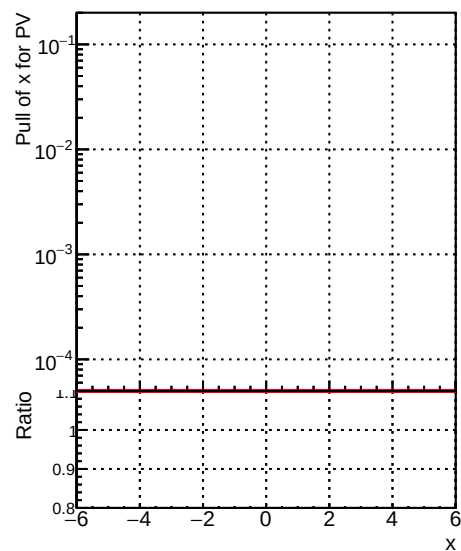
RecoPVAssoc
