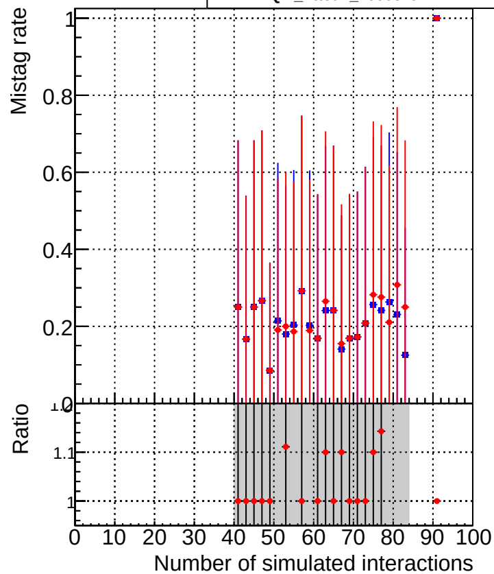
■ DQM_original_1000evt ● DQM_fitted4_1000evt
