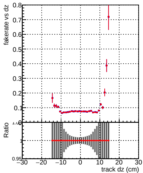
Fake rate vs dz — DQM_original_1000evt — DQM_fitted4_1000evt
