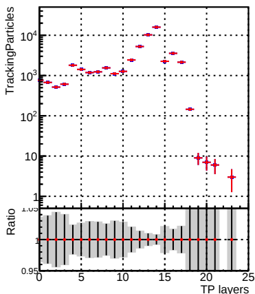
N of sim — DQM_fitted4_1000evt
