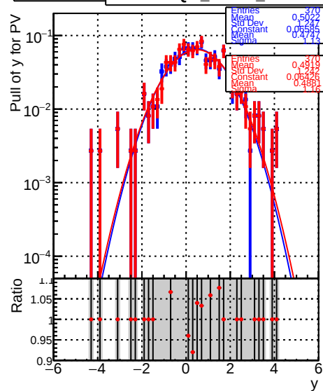
Legend: — DQM_original_1000evt — DQM_fitted4_1000evt
