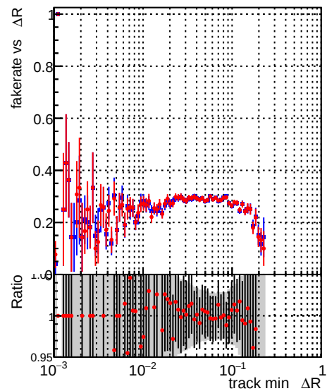
—•— DQM_original_1000evt —•— DQM_fitted4_1000evt
