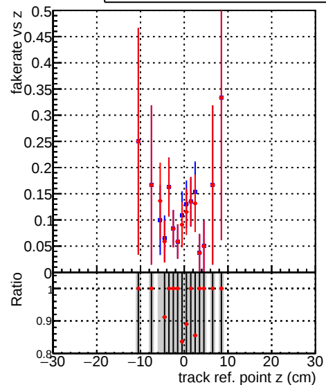
Fake rate vs —●— DQM_original_1000evt —●— DQM_fitted4_1000evt
