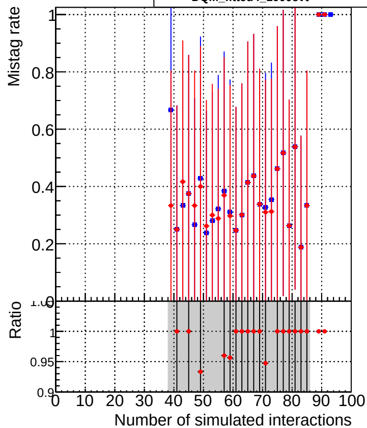
■ DQM_original_1000evt ● DQM_fitted4_1000evt
