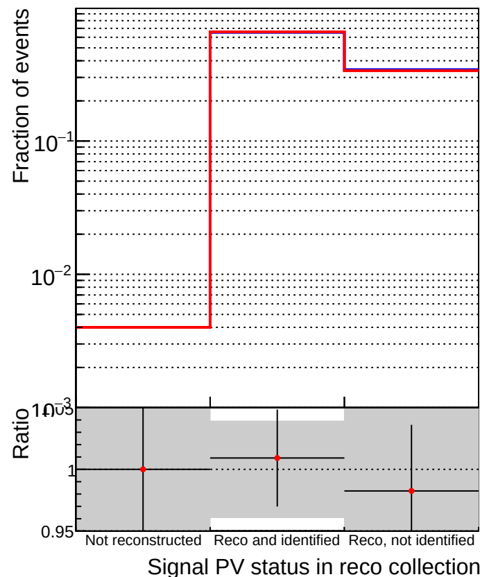
■ DQM_original_1000evt ● DQM_fitted4_1000evt
