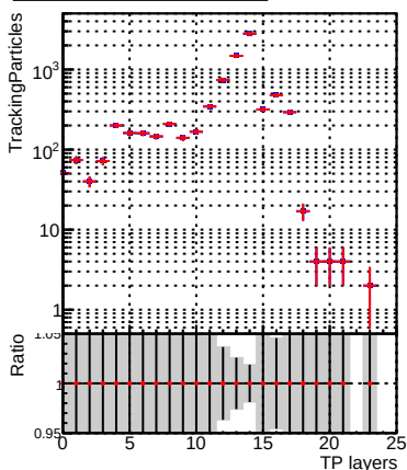
—●— DQM_fitted4_1000evt
