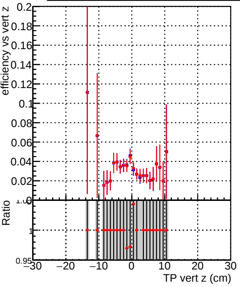
Efficiency vs vertpos Legend: DQM_original_1000evt DQM_fitted4_1000evt
