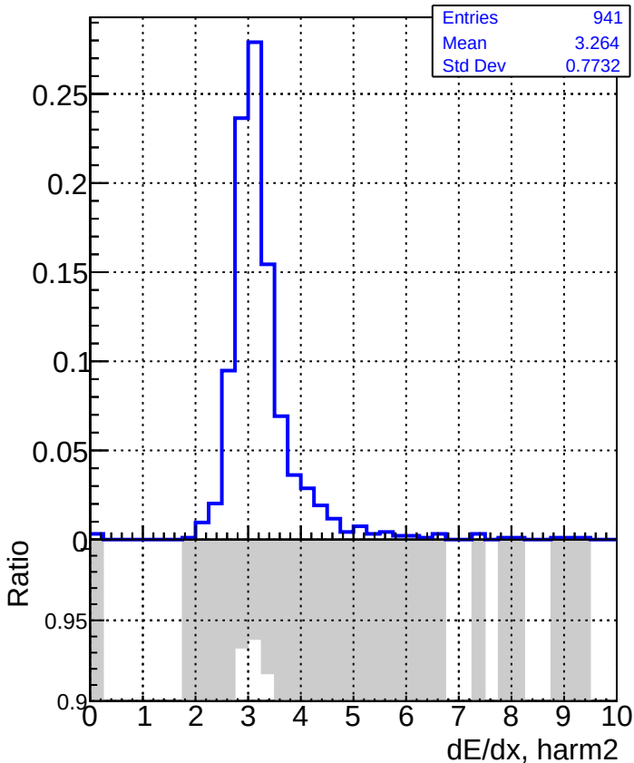
dE/dx estimator 1
