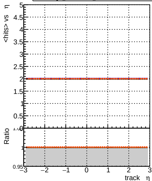
mean hits — DQM_CKFFit_1000evt — DQM_CKFREFit_1000evt — DQM_MkFitREFit_1000evt — DQM_TESTOLHIT_POS
