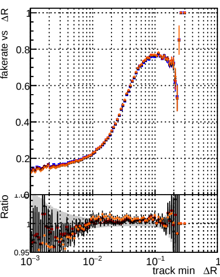
Fake rate vs \Delta R (track, jet) Legend: - DOM CKFEE fit 1000evt - DOM CKFEE fit 1000evt - DOM CKFEE fit 1000evt - DOM CKFEE fit 1000evt
