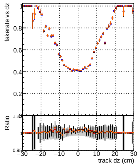
Fake rate vs dz — DOM CKFIT 1000evt — DOM CKFIT 1000evt — DOM TESTOFT 100evt
