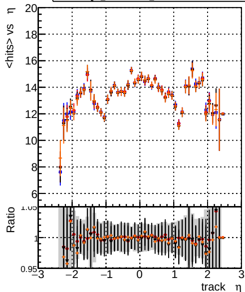
DOM_CKFFit_1000evt DOM_CKFREFit_1000evt DOM_MkFitREFit_1000evt DOM_TESTOLHIT_POS mean hit
