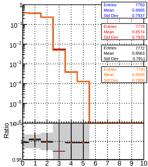
mean hits DOM_CKFFit_1000evt DOM_CKFREFit_1000evt DOM_MkFitREFit_1000evt DOM_TESTOLHIT_POS
