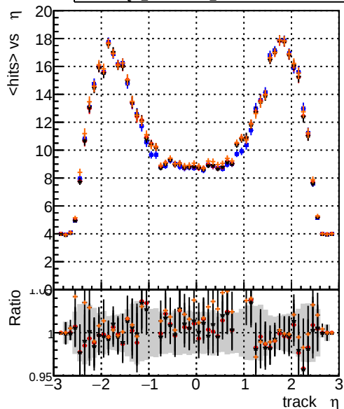
mean hit DOM_CKFFit_1000evt DOM_CKFREFit_1000evt DOM_MkFitREFit_1000evt DOM_TESTOLHIT_POS
