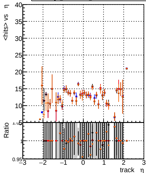
mean hits vs \eta DOM_CKFFit_1000evt DOM_CKFREFit_1000evt DOM_MkFitREFit_1000evt DOM_TESTOLHIT_POS
