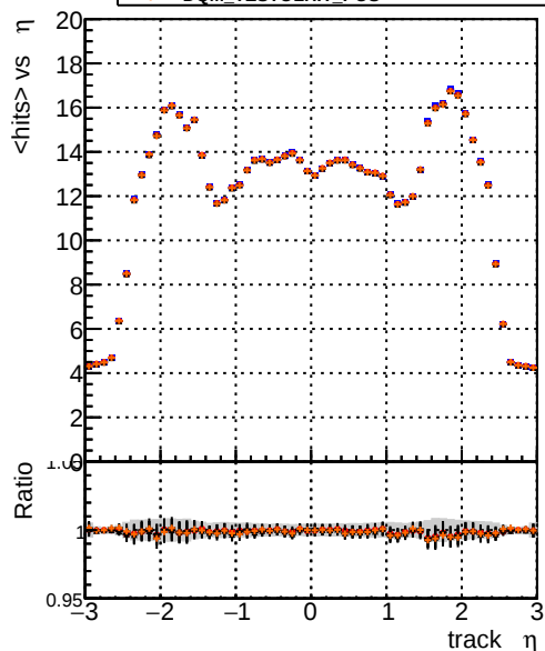
mean hits DOM_CKFFit_1000evt DOM_CKFREFit_1000evt DOM_MkFitREFit_1000evt DOM_TESTOLHIT_POS
