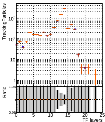
—●— DQM_MkFitREFit_1000evt —●— DQM_TESTOLHIT_POS
