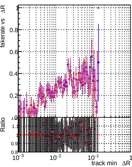
Fake rate vs \Delta R(\text{track, jet}) DOM CKFEE CKFEE+1000evt CKFEE+1000evt+1000evt CKFEE+1000evt+1000evt+1000evt TEST
