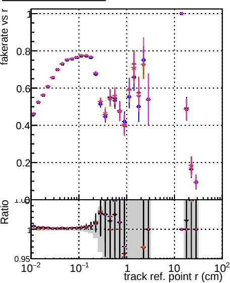
Fake rate vs DOM-CKEFit-10000vt DOM-CKEFit-1000vt DOM-CKEFit-10000vt DOM-TESTOLHIT-10000vt-50000t
