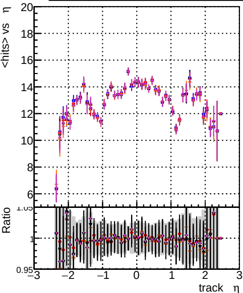
mean hits vs \eta DOM CKFEEIT 1000evt DOM CKFEREEL 1000evt DOM MCFEEIT 1000evt DOM TESTOLHIT 1000evt DOM TESTOLHIT 1000evt-50000t
