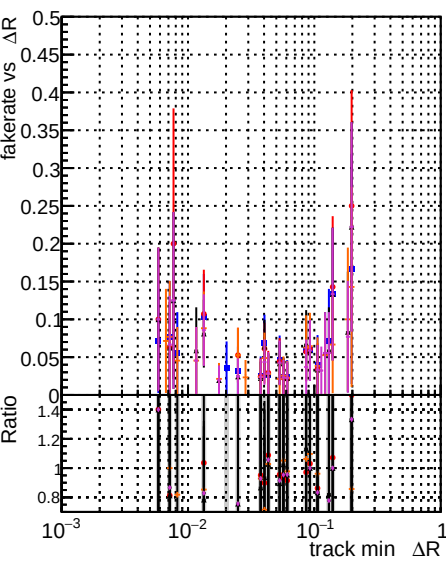
Fake rate vs ΔR(track, jet) Legend: DOM CKFit 1000evt DOM CKFit 10000evt DOM CKFit 100000evt DOM TEST OHIT 1000evt DOM TEST OHIT 10000evt DOM TEST OHIT 100000evt
